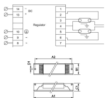
Technische Daten Philips HF-R 258 TL-D EII 220-240V für 2x58W
